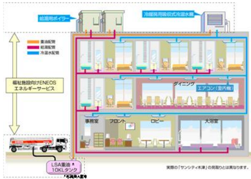
「サンシティ木津」の冷暖房・給湯設備概要
